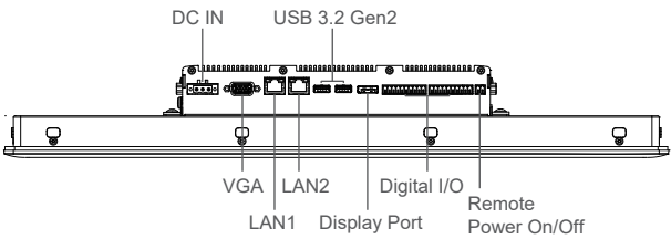
Right I/O
