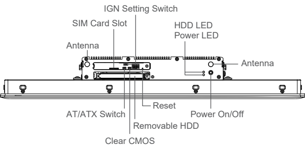
Left I/O
