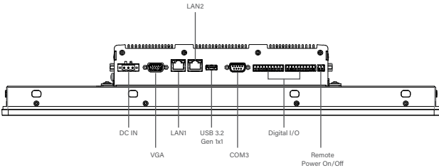
Right I/O
