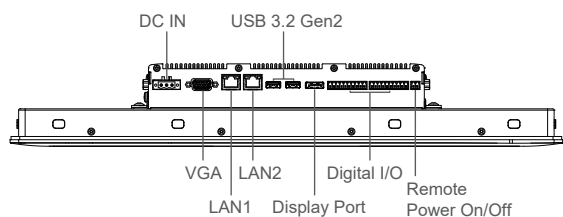
Right I/O
