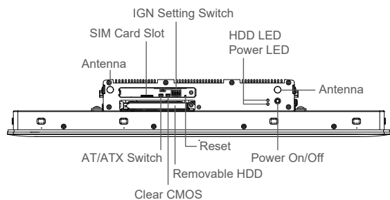
Left I/O
