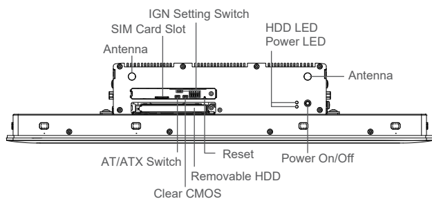
Left I/O
