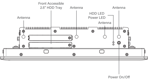
Left I/O
