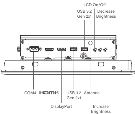
Right I/O
