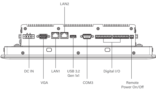
Right I/O
