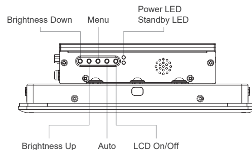
Right I/O
