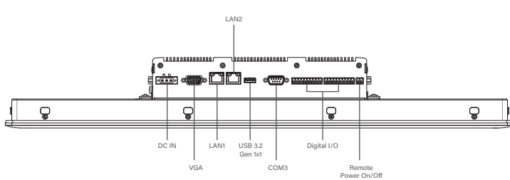
Right I/O
