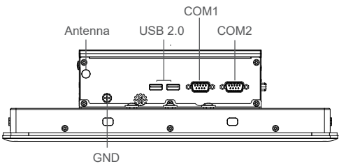
Left I/O
