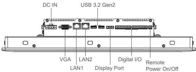
Right I/O
