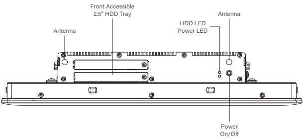
Left I/O
