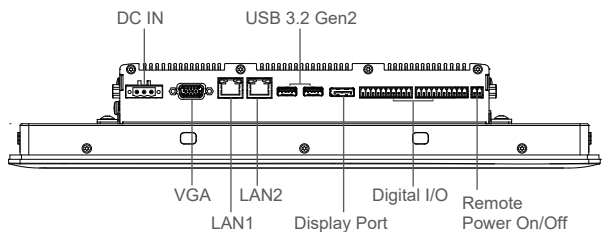
Right I/O
