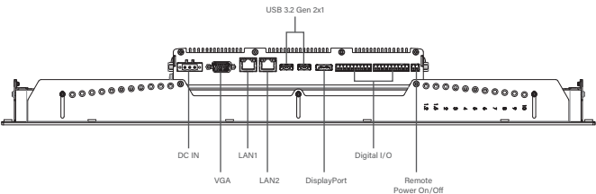
Right I/O
