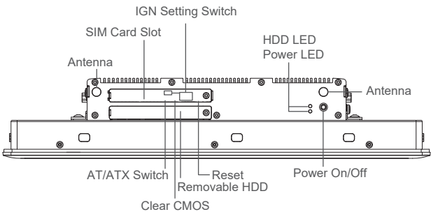
Left I/O
