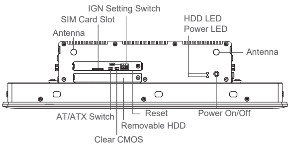
Left I/O
